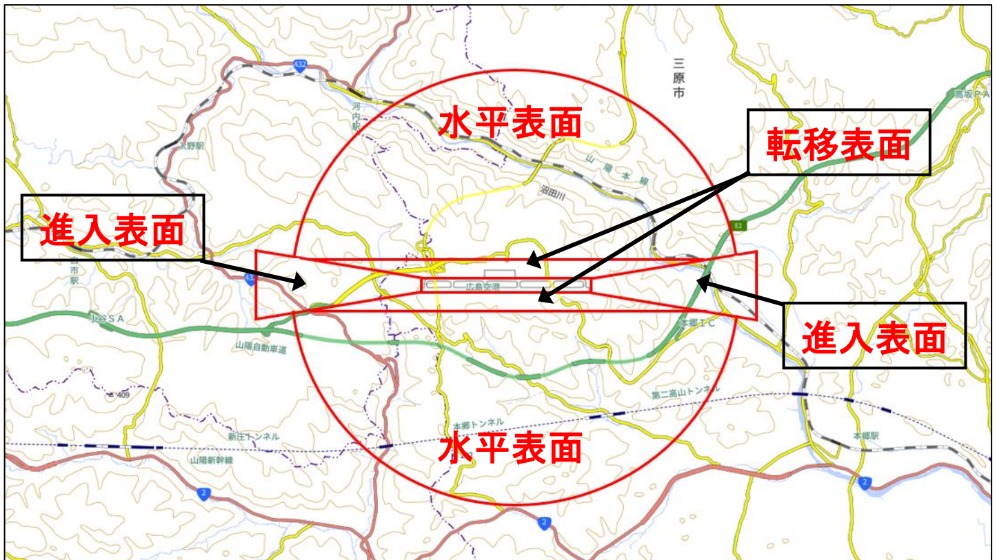
広島空港の制限表面区域図
